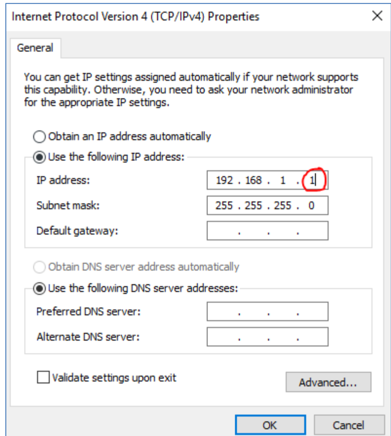
Slika 29: Promjena IP adrese računala i unos "subnet mask"
