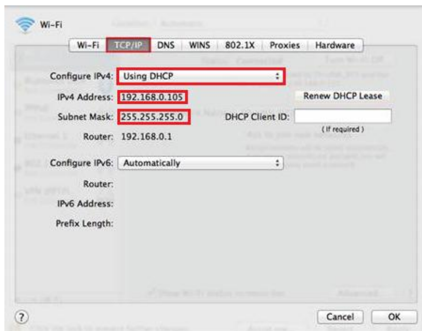
Slika 33: Promjena mrežnih postavki
