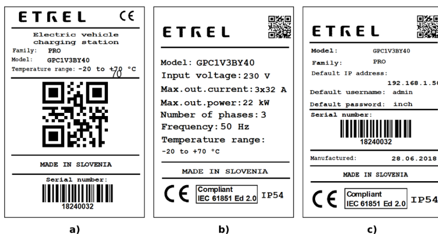
Slika 8: Tri različite naljepnice, na pakiranju, na servisnim vratašcima i unutar prostora za održavanje, iza servisnih vratašca
