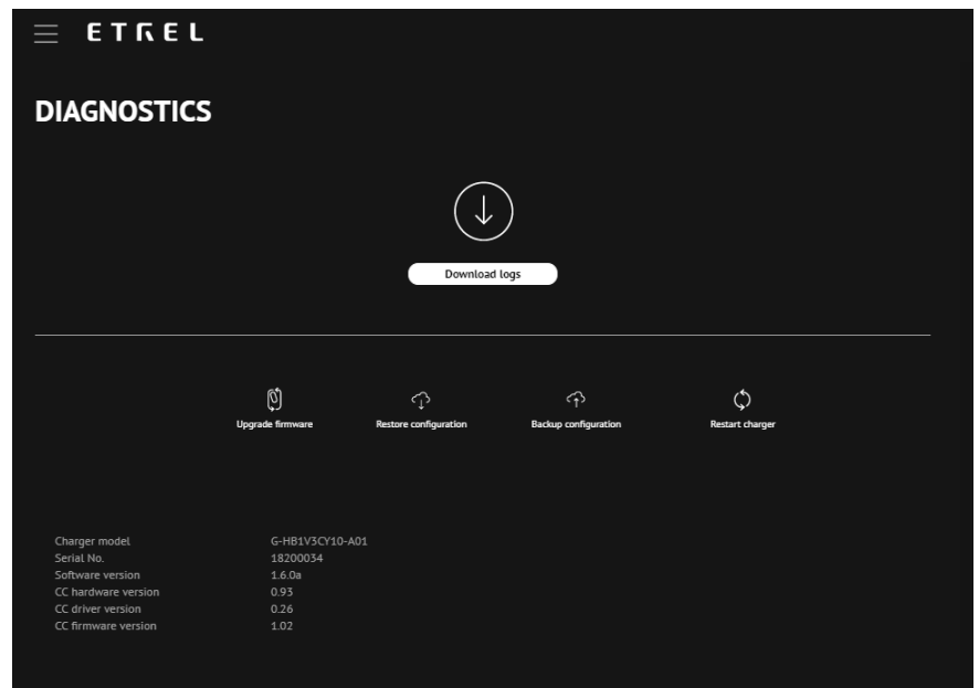
Slika 35: Dijagnostika na mrežnom sučelju
