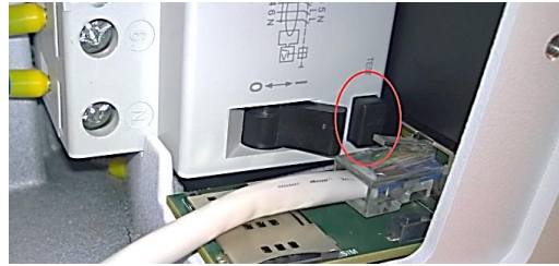
Slika 39: Gumb za testiranje FID sklopke (RCD)
