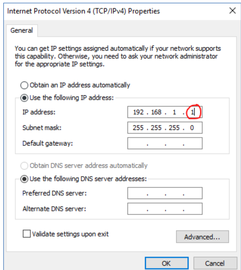
Slika 29: Spreminjanje IP naslova računalnika in vpis "subnet mask"
