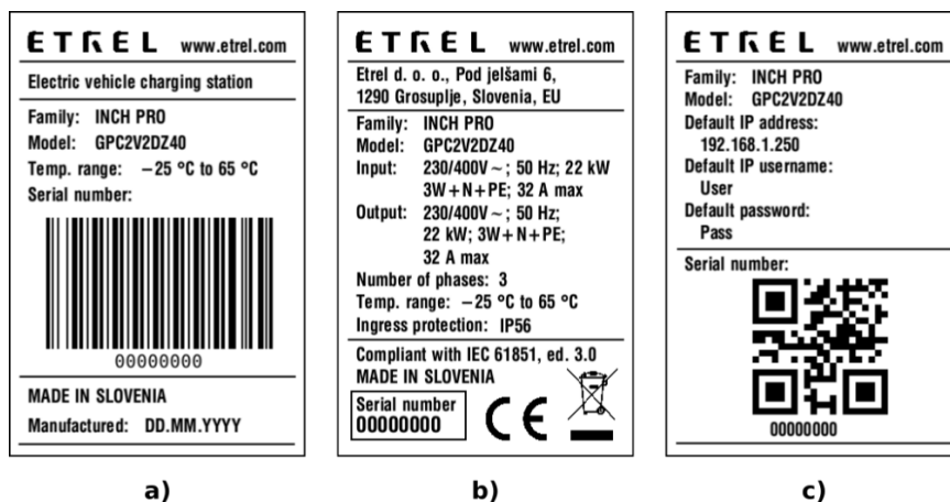
Slika 8: Tri različne nalepke, na embalaži, na servisnih vratcih in znotraj vzdrževalnega prostora, za servisnimi vratci
