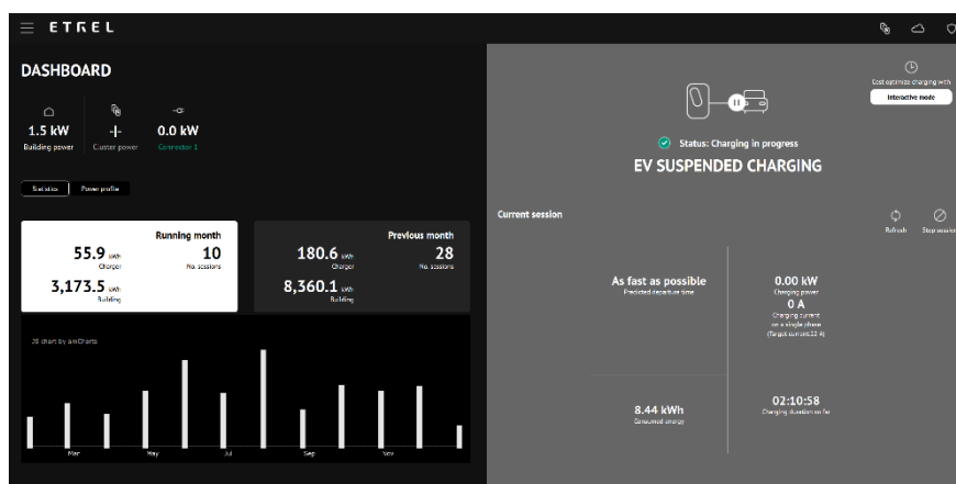
Figur 39: Information om aktuell session som visas i webbgränssnittet
