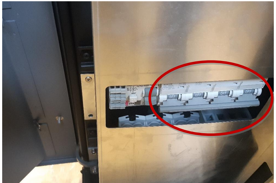
Figur 45: Huvudströmbrytaren kan användas för att återställa laddningsstationen
