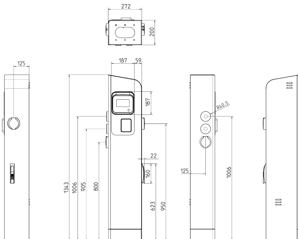
Figur 5: INCH Duo-mått på modeller med uttagshöjder enligt PAS 1899
