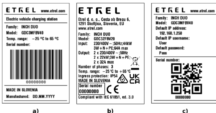
Figur 9: Tre olika klistermärken på laddningsstationen
