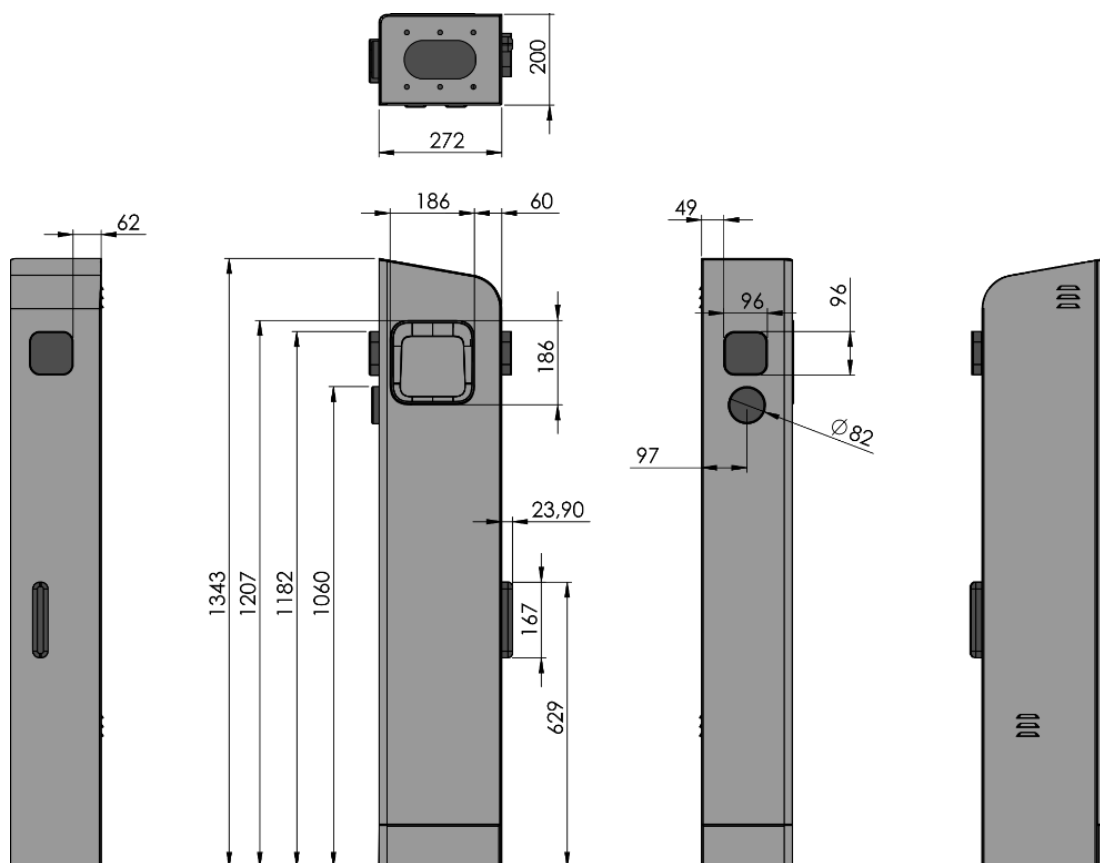
Figur 4: INCH DUO-laddningsstationens mått
