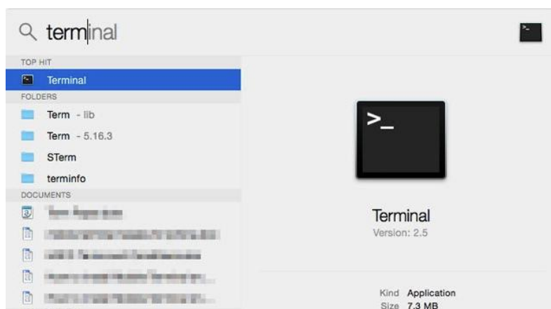
Figur 29: Kör Terminalprogramvaran
