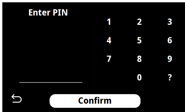
Figur 13: Ange PIN-kod
