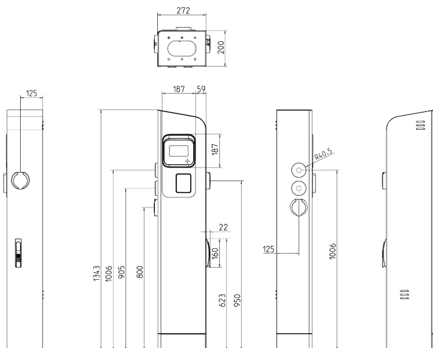
Slika 5: Dimenzije modelov polnilnih postaj INCH Duo z višino vtičnic v skladu s PAS 1899
