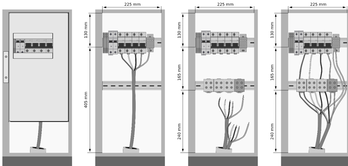
Slika 6: Prikaz napajalnega predela
