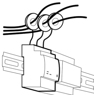
Slika 8: Load Guard
