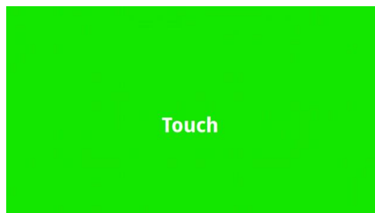
Slika 10: Ohranjevalnik zaslona
