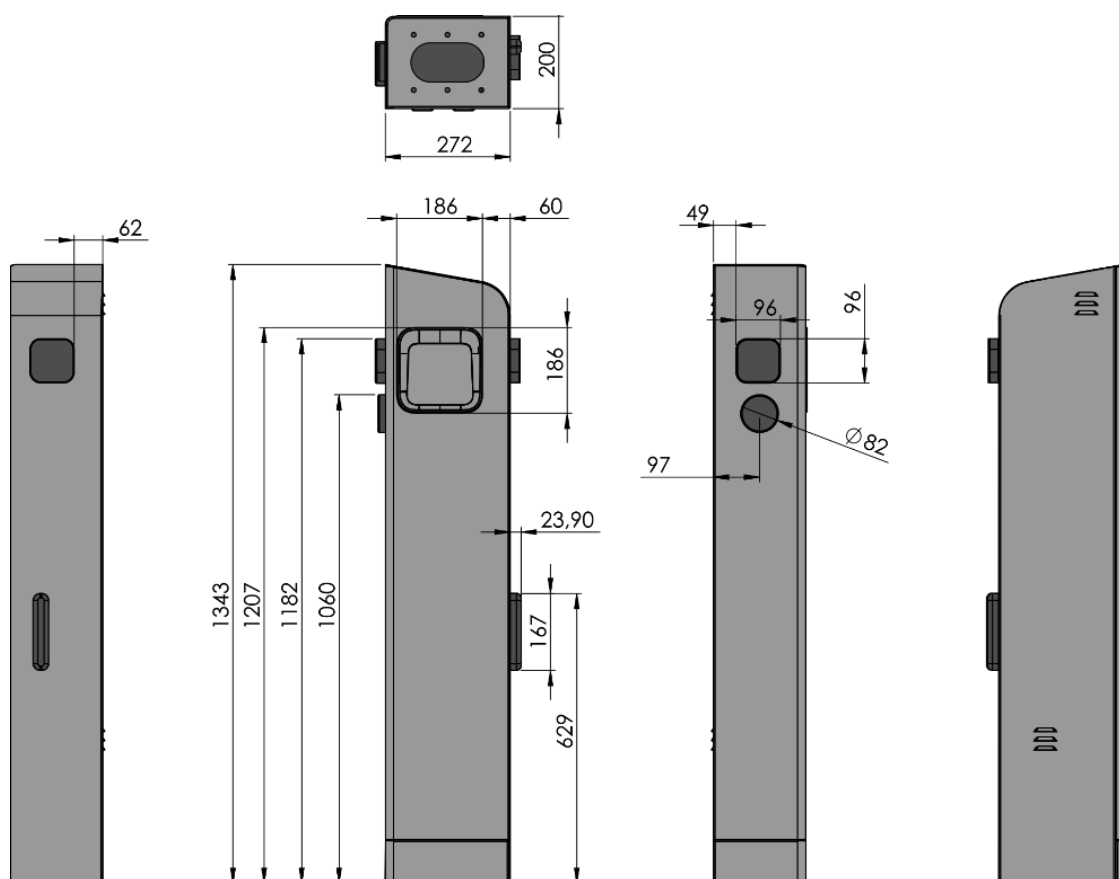
Figura 4: Dimensões da estação de carregamento INCH DUO
