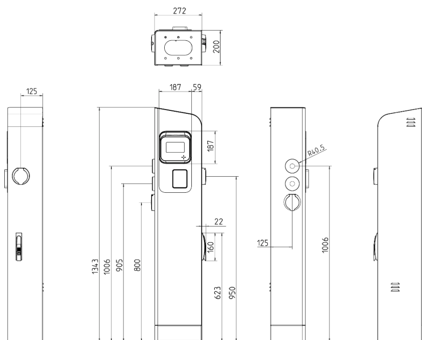
Figura 5: INCH Duo dimensões dos modelos com alturas de tomada de acordo com PAS 1899
