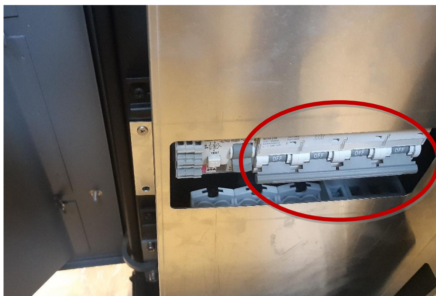
Figura 45: O disjuntor principal pode ser utilizado para reiniciar a estação de carregamento
