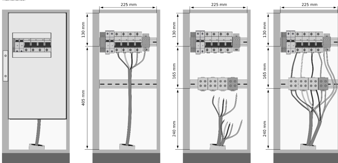
Figura 6: Dimensões do compartimento da fonte de alimentação do INCH DUO
