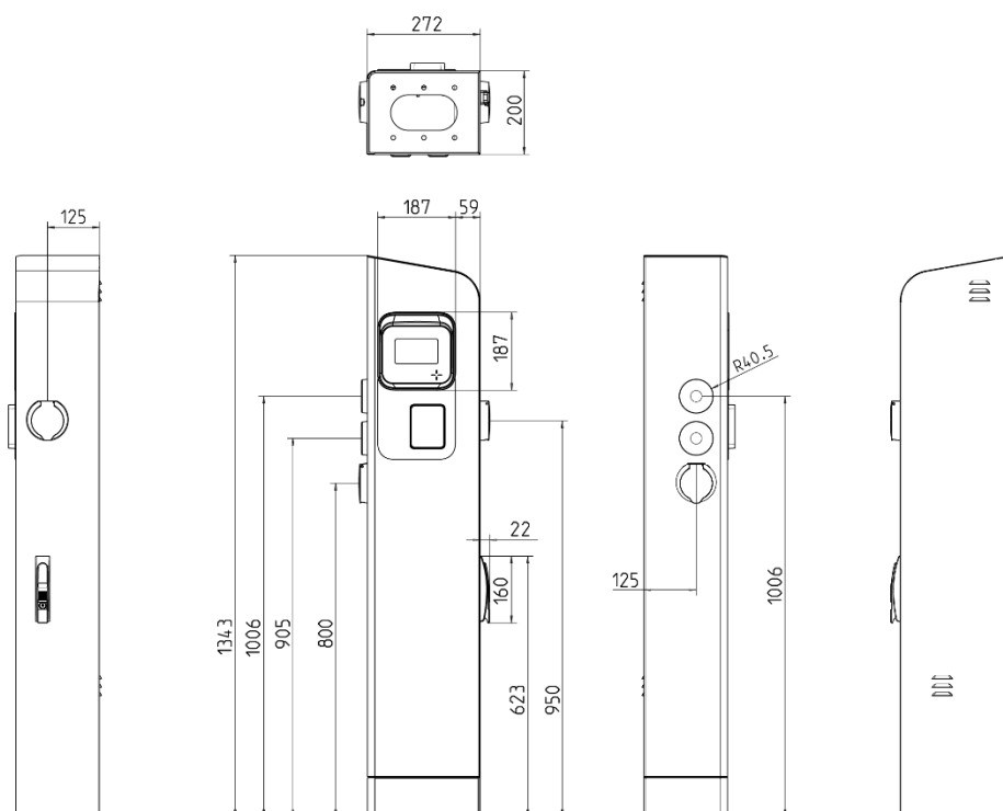
Rysunek 5: INCH Duo wymiary modeli z gniazdami o wysokości zgodnej z PAS 1899
