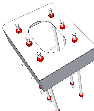
Rysunek 7: Podziemny element kotwiący
