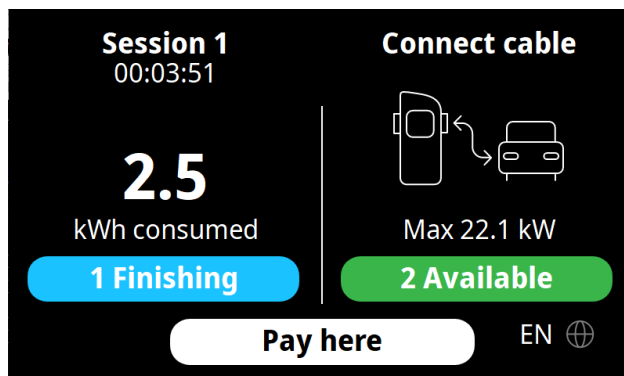
Rysunek 20: Przykład stanu wyświetlanego na ekranie LCD
