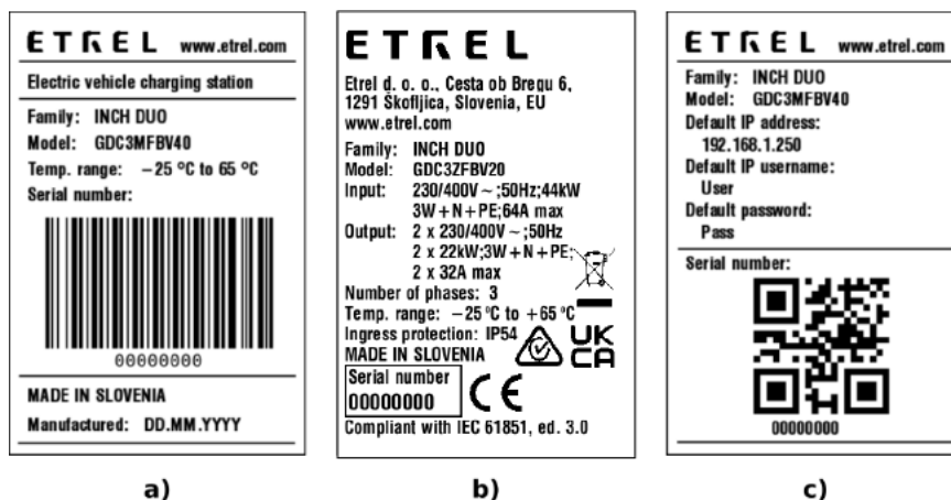
Rysunek 9: Trzy różne naklejki stacji ładowania
