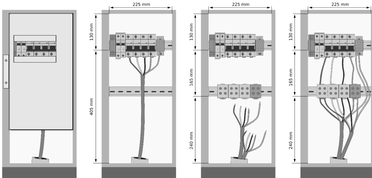
Rysunek 6: Wymiary komory zasilania INCH DUO
