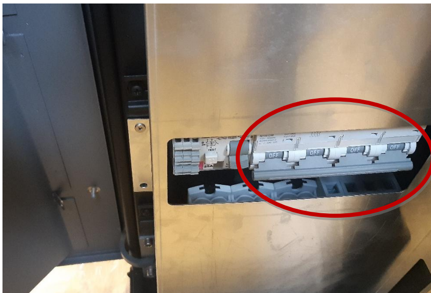
Rysunek 45: Główny wyłącznik automatyczny może służyć do resetowania stacji ładowania
