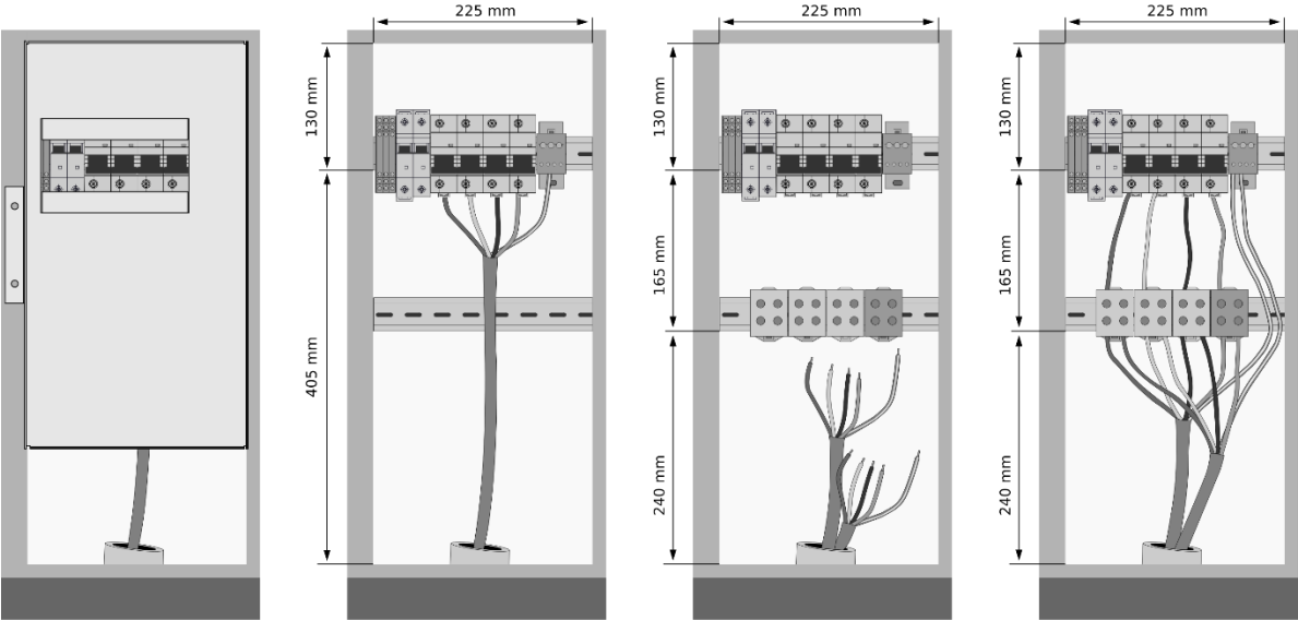
Figure 6: Dimensions du boîtier d'alimentation électrique de la borne INCH DUO
