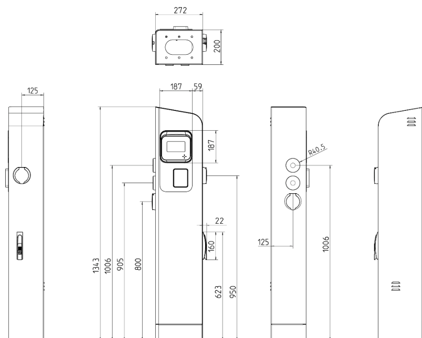
Figure 5: Dimensions INCH Duo des modèles avec hauteurs de prises conformes à PAS
