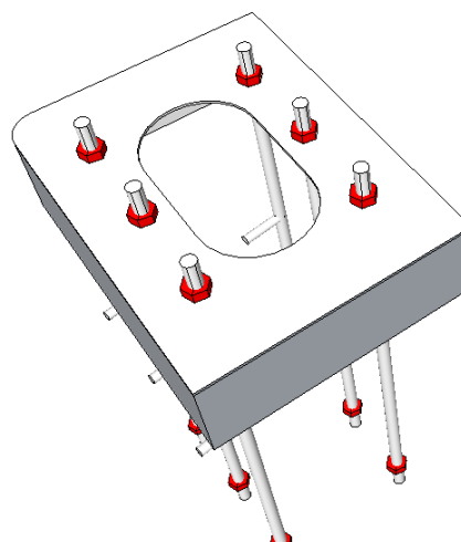
Figure 7: Élément d'ancrage enterré
