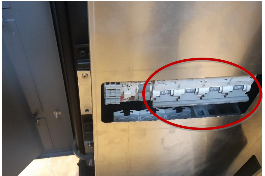
Figure 45: Le disjoncteur principal peut être utilisé pour réinitialiser la station de charge
