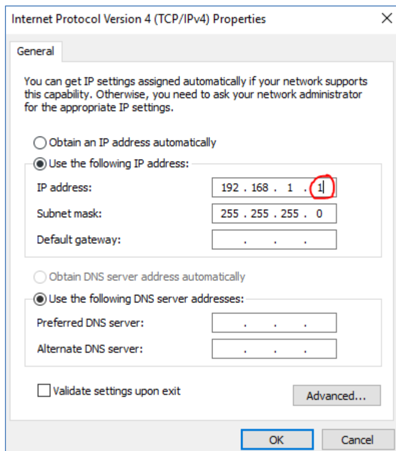
Figure 33: Modifiez l'IP de l'ordinateur et le masque de sous-réseau
