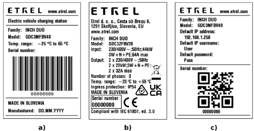
Figure 9: Les trois autocollants de la station de charge
