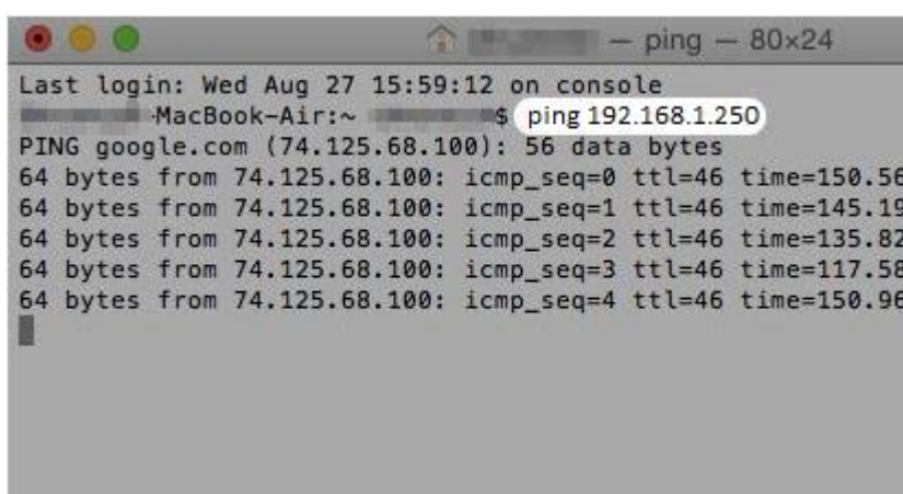
Figur 30: Ping ladestationen ved at skrive ping og ladestationens IP
