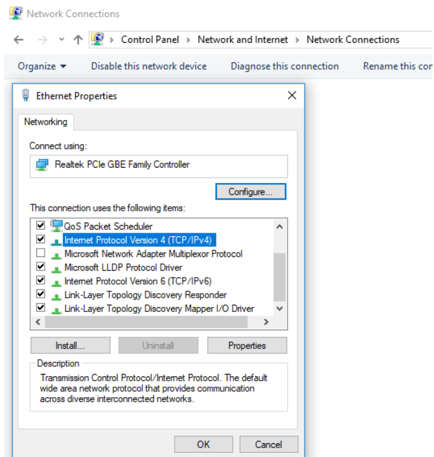
Figur 32: Find TCP/IPv4 (Internet Protocol Version 4) i netværksegenskaberne
