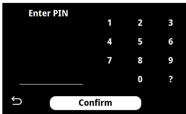
Figur 13: Indtast PIN-kode
