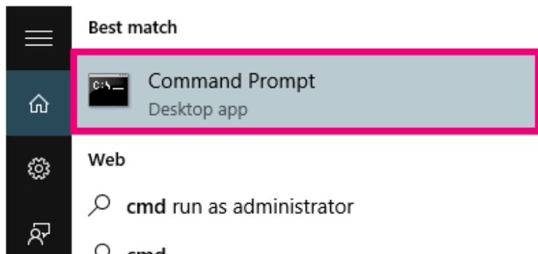
Figur 27: Åbn kommandoprompt
