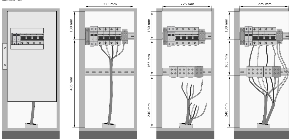
Figur 6: Dimensioner på INCH DUO-strømforsyningsrummet
