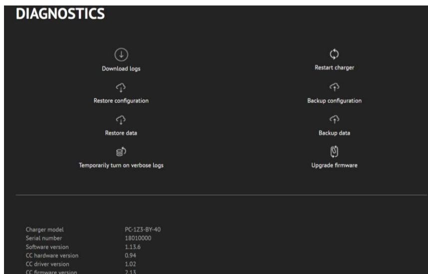
Figur 41: Diagnosticering webgrænseflade-modul
