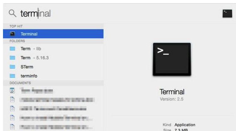
Figur 29: Kør Terminal-appen
