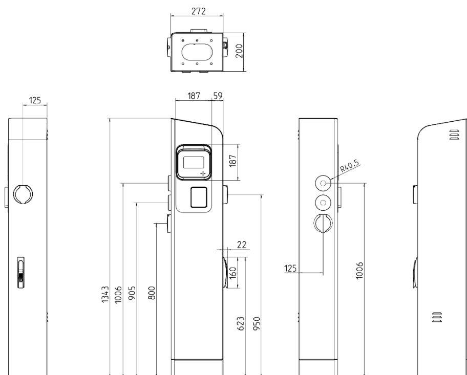
Figur 5: INCH Duo-mål på modeller med stikkontakthøjder i henhold til PAS 1899
