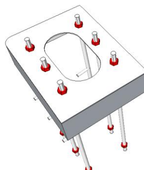
Figur 7: Underjordisk forankringselement
